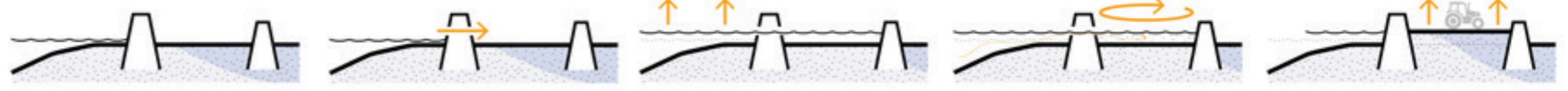
dubbele dijk gebruik maken van bestaande dijken openen opening in buitenste zeewering getijdeninvloed zeewater stroomt de wisselpolder in tijdens hoogtij sedimentaanvoer de getijdendynamiek vervoert sediment de wisselpolder in meegroeien de wisselpolder creëert natuurlijk opgehoogd land dat meegroeit met zeespiegelstijging
