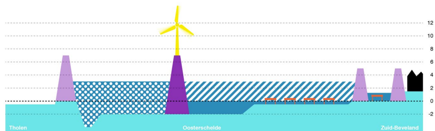
DOORSNEDE OVER DE OOSTERSHELDE
