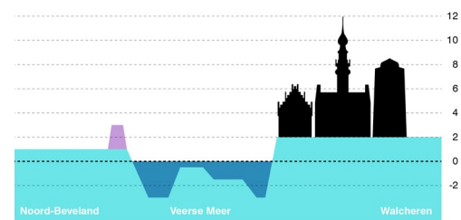
DOORSNEDE VEERSE MEER TER PLATSE VAN VEERE
