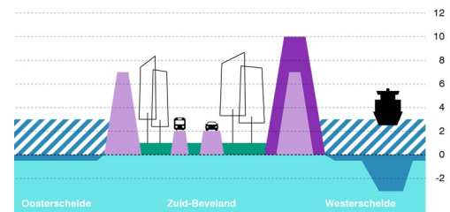
DOORSNEDE OVER DE HALS VAN MIDDEN ZEELAND
