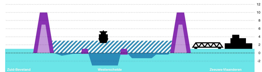
DOORSNEDE OVER DE WESTERSCHELDE TER PLAATSE VAN TERNEUZEN
